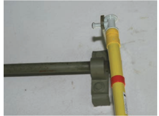
Erottimen ohjaaminen IS SK -eristys-sauvalla ja SSK -käyttöpäällä.
