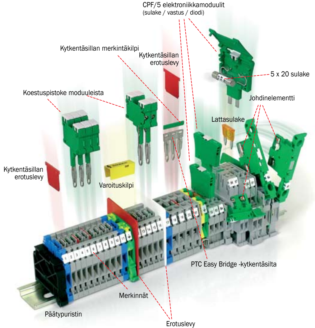
CBC Sarjan riviliittimet ja niihin sopivat tarvikkeet
